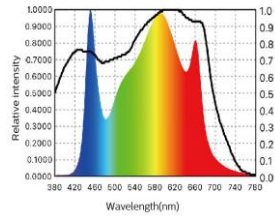
植物灯光谱/003
